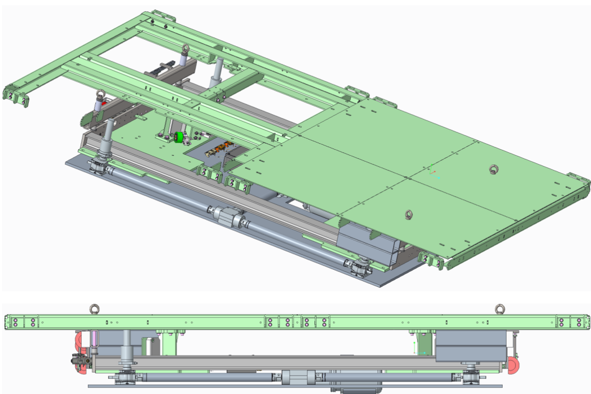
Schnitt des optimierten System mit neuem Antrieb
