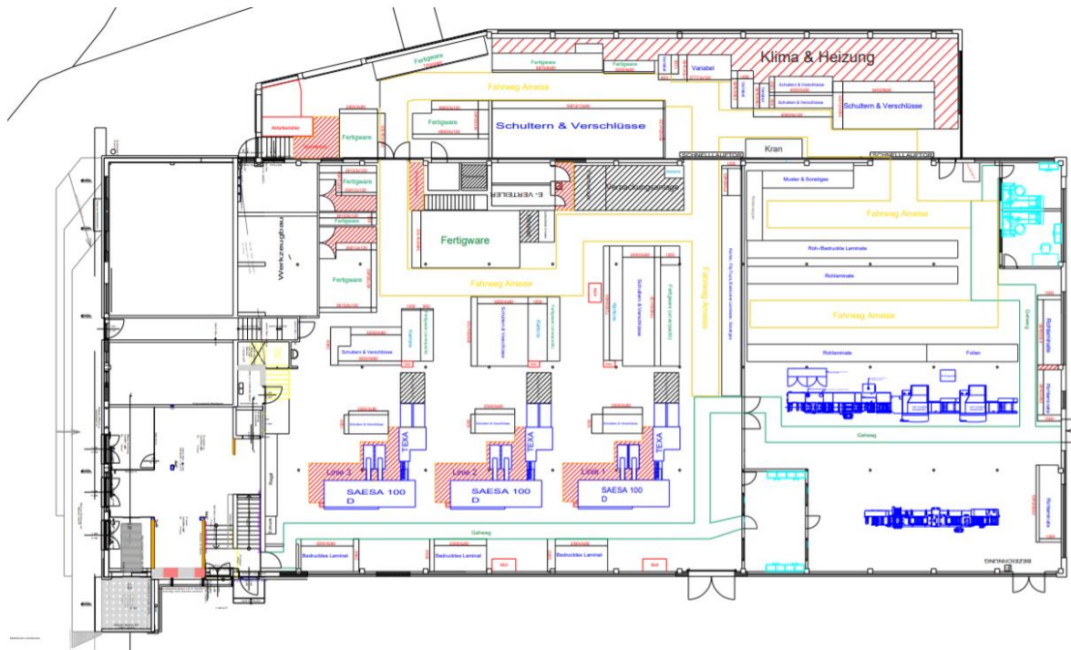
Fertig konzipierter digitaler Gebäudegrundriss
